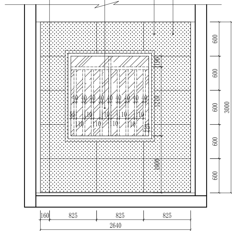
ELEVATION SCALE 1:100 纪检工作室C立面图
