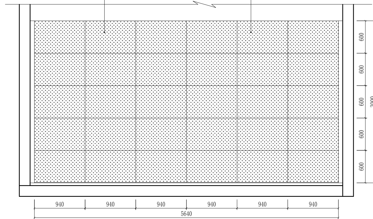
ELEVATION SCALE 1:100 纪检工作室D立面图
