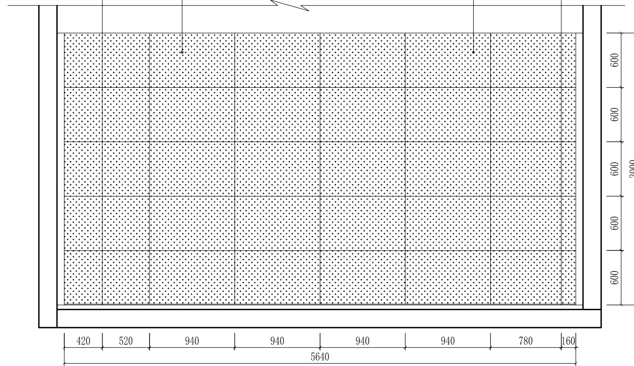
ELEVATION SCALE 1:100 纪检工作室B立面图
