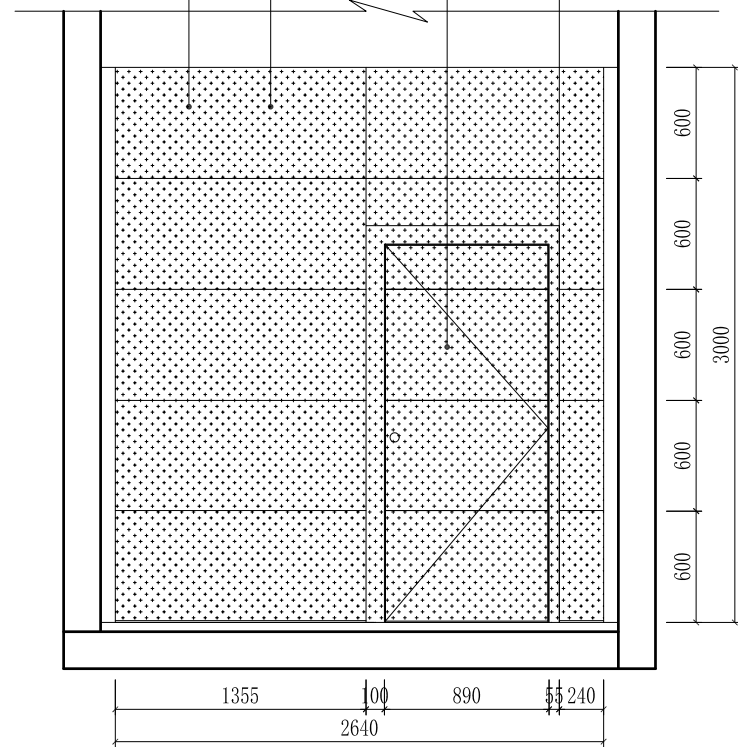
ELEVATION SCALE 1:100 纪检工作室A立面图
