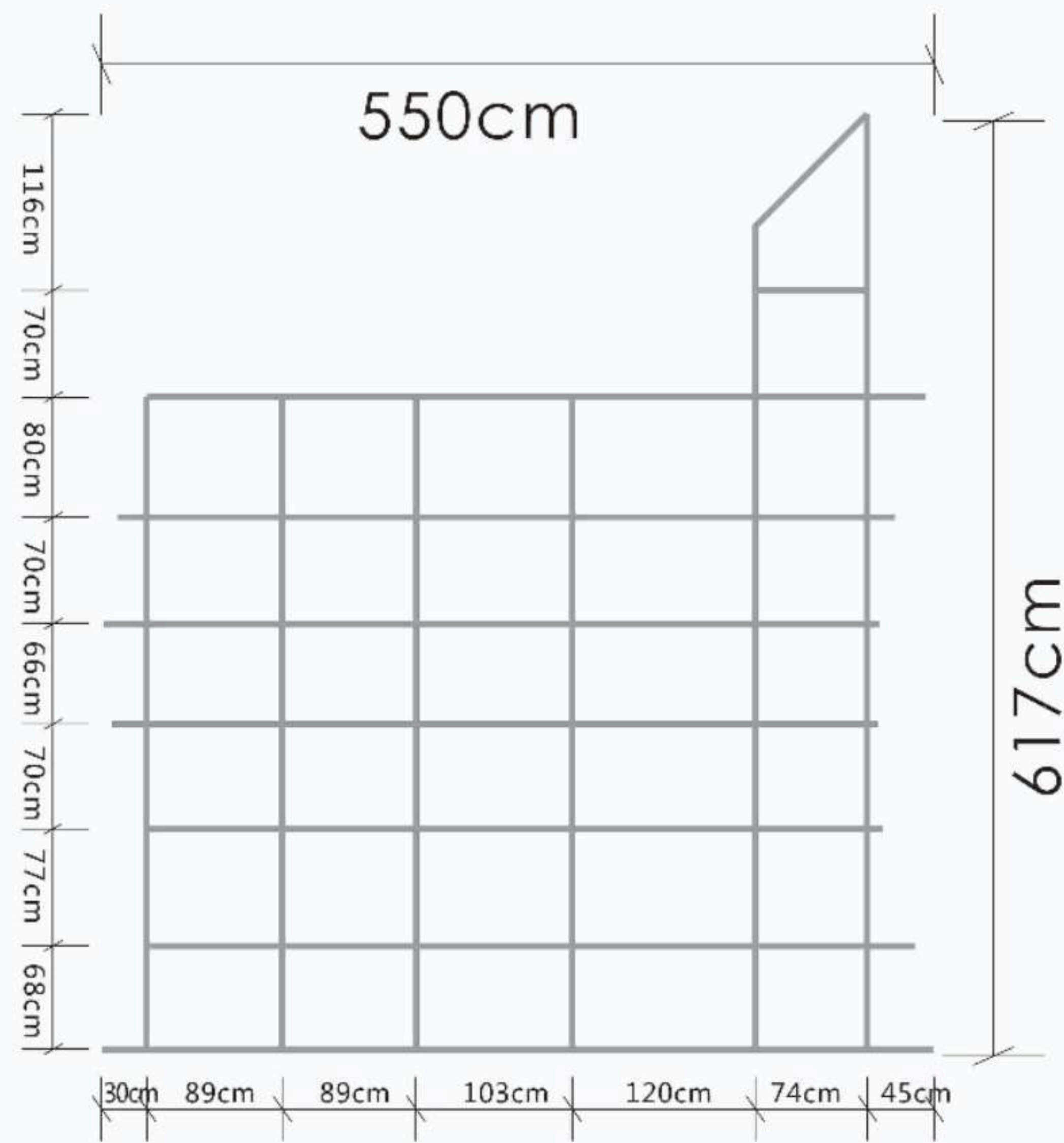
Ⓐ 5#镀锌角铁钢架结构示意图
