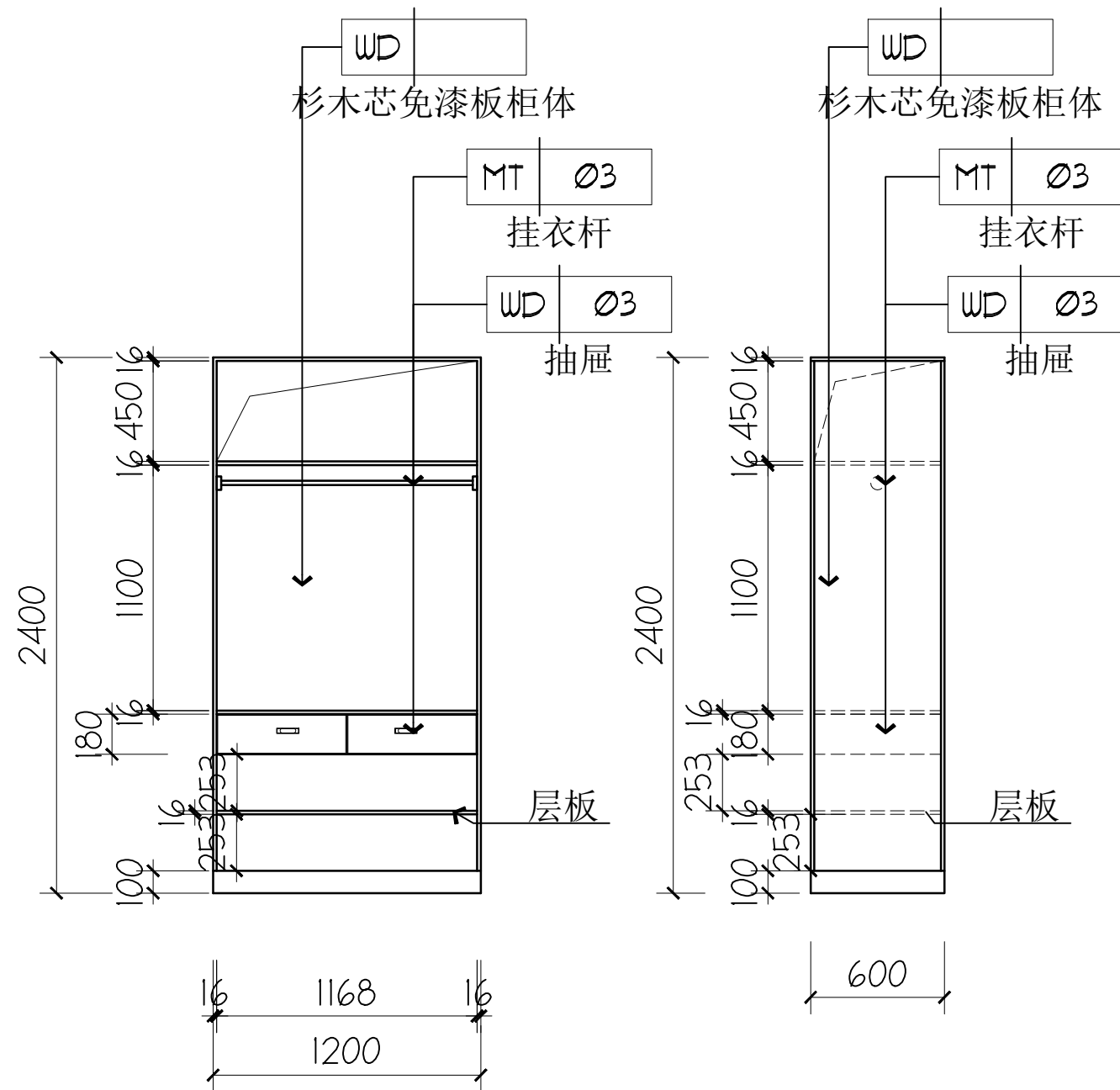
柜体尺寸图
